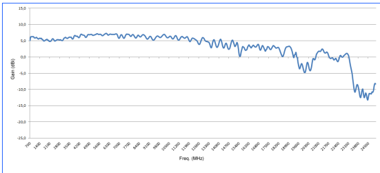
Diagrama de ganancia HyperLOG 60250
