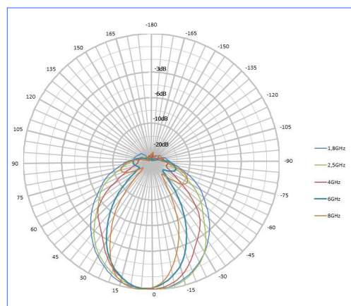
Patrón vertical Línea HyperLOG 60xxx
