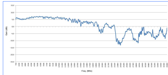
Diagrama de ganancia HyperLOG 60350
