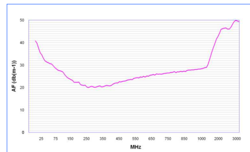
Factor de antena BicoLOG 20300
